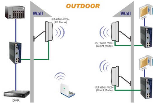
AP-Client Mode
